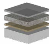
Recubrimiento Stonhard (opcional) Stonclad (Mortero) Imprimación Stonhard Sustrato
